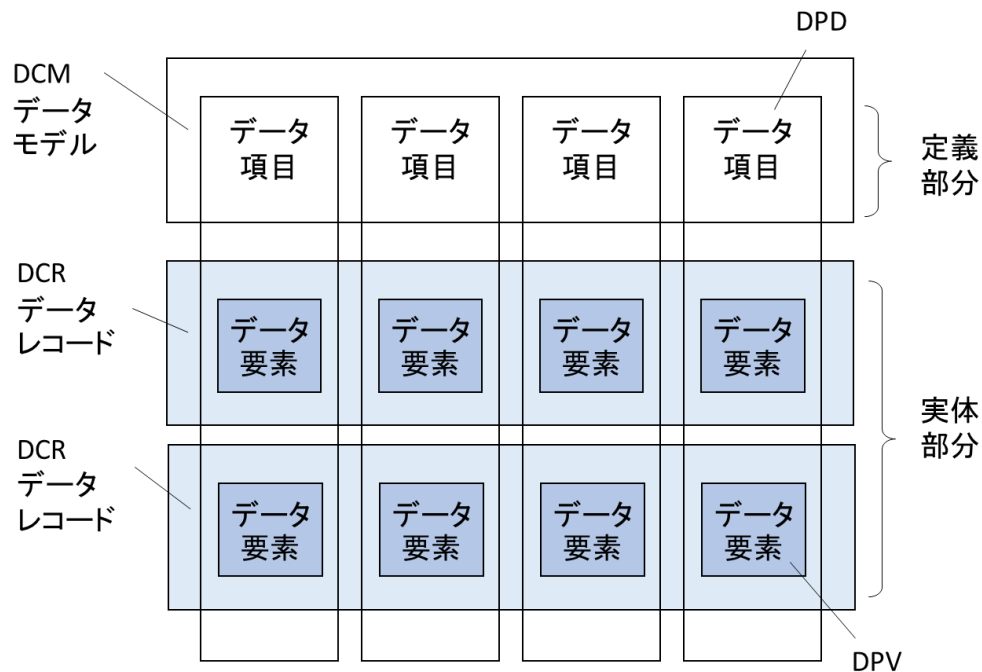
図 11 モデルと実体の関係
