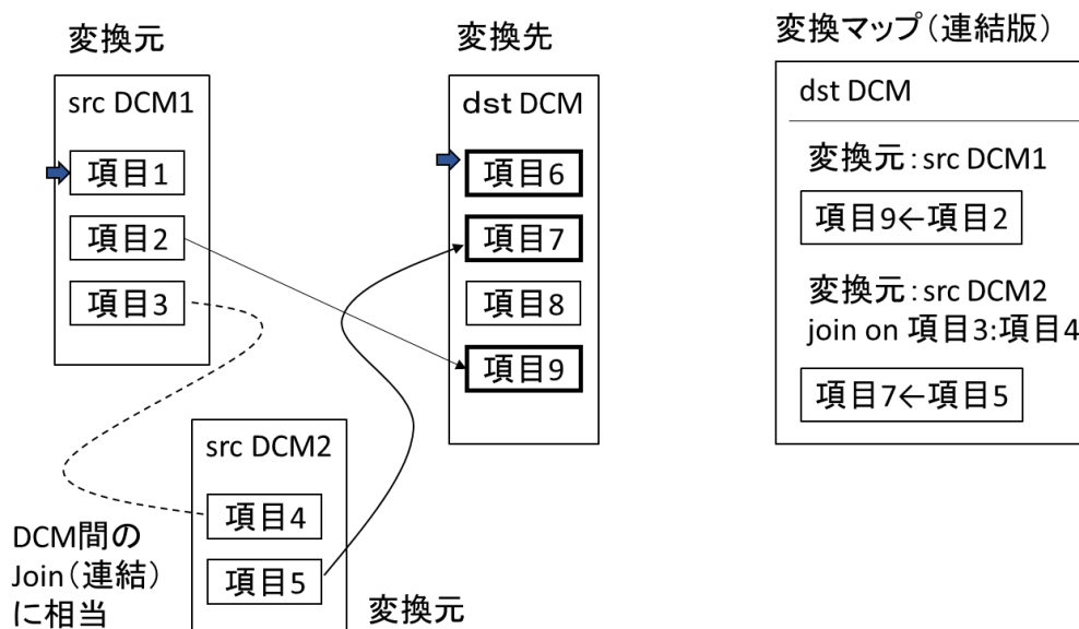
図 25 マッピング (1対多の場合)
