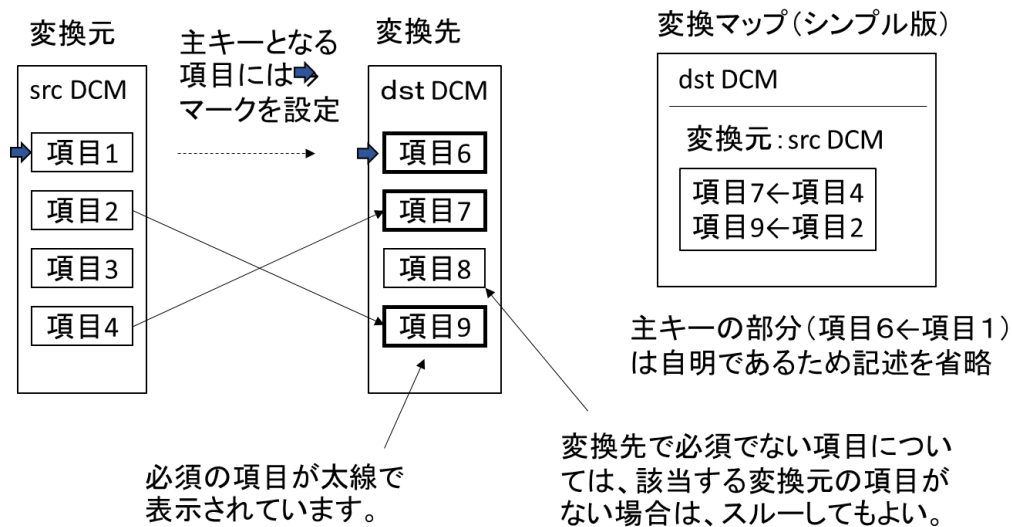
図 24 マッピング (1対1の場合)
